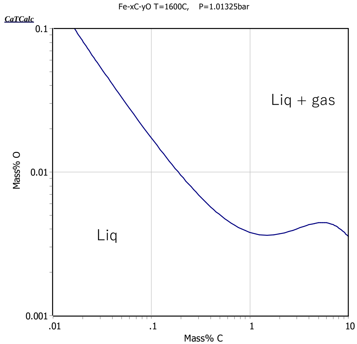
Fe-C-O 3 元系 1600°C等温断面图 Solubility of oxygen in molten Fe-C
